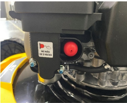
Primer bulb and fuel-system inspection.
